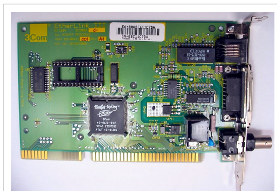
Tarjeta de red ISA de 10 Mbps con conectores RJ-45, AUI y 10Base2.
